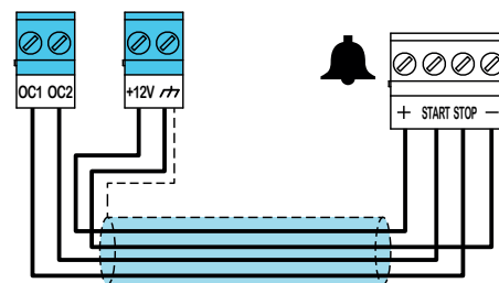
Collegamento a 4 fili
