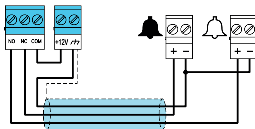
Collegamento a 3 fili
